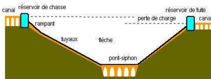
Fig2.24.a : schéma d'un pont-siphon.
