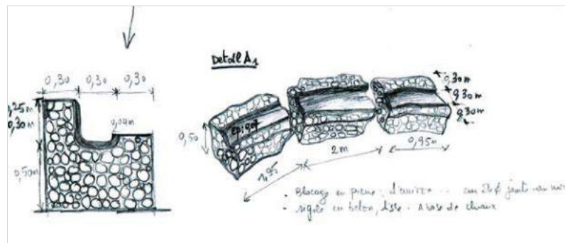
Fig 4.39 : Schématisation des 03 segments du point 15 (A.1) propriété Khoudir
