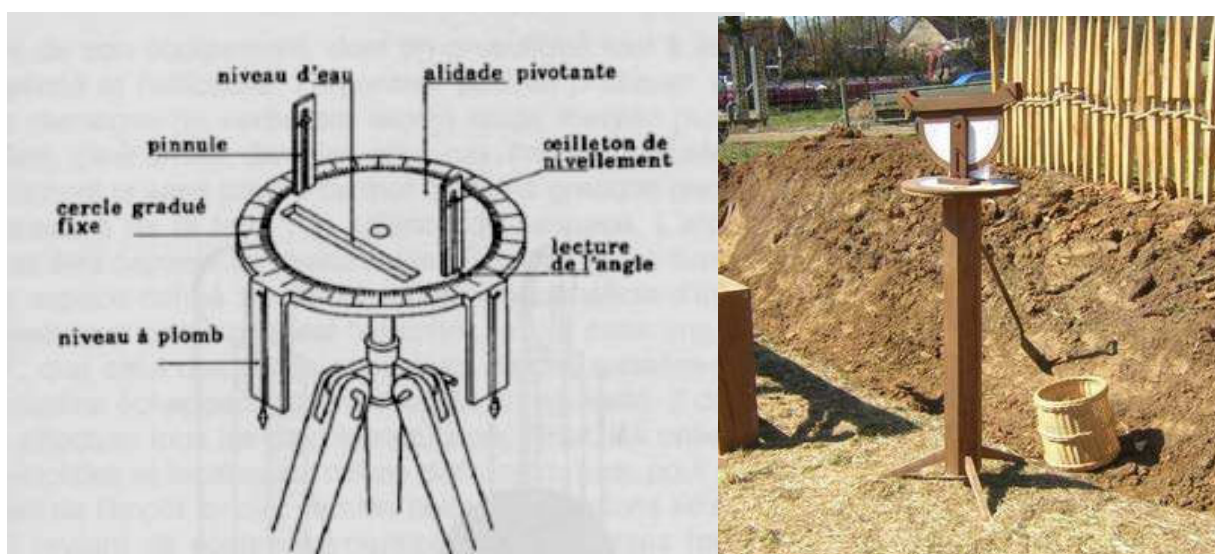
Fig 1 : vue et plan du dioptré
