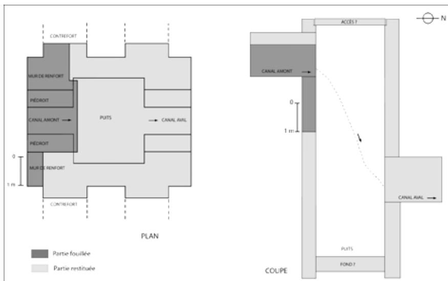
Fi. 2.15 : Plan et coupe du puits de rupture de pente de la cascade de l'aqueduc de Montjeu
