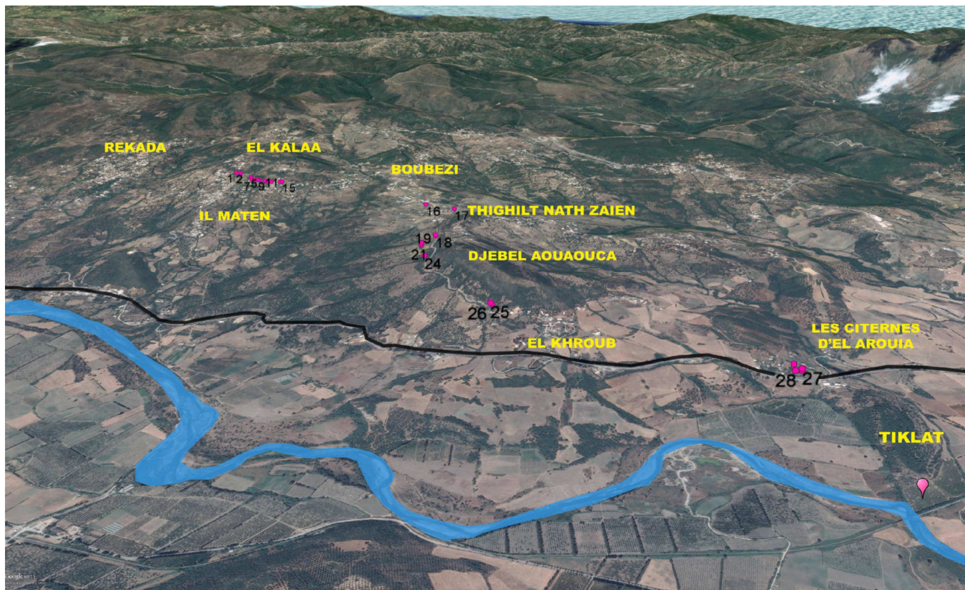
Fig 4. 29: repérage des points relevés des vestiges de l'aqueduc sur Image aérienne Source : Auteurs
