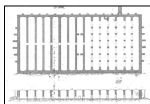
Fig. 2.9 : type de citernes à Tiklat ou Hippone
