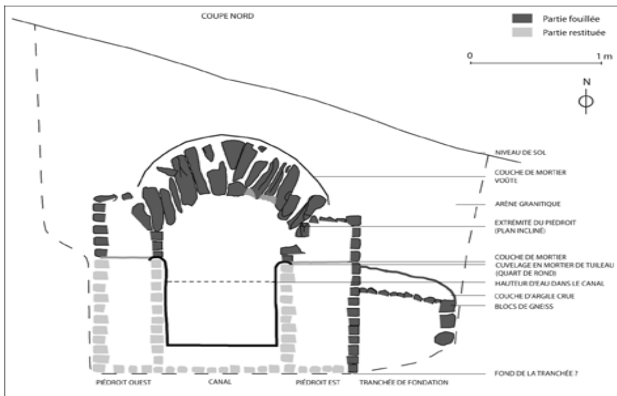
Fig. 2.16 : coupe schématique sur un aqueduc semi enterré
