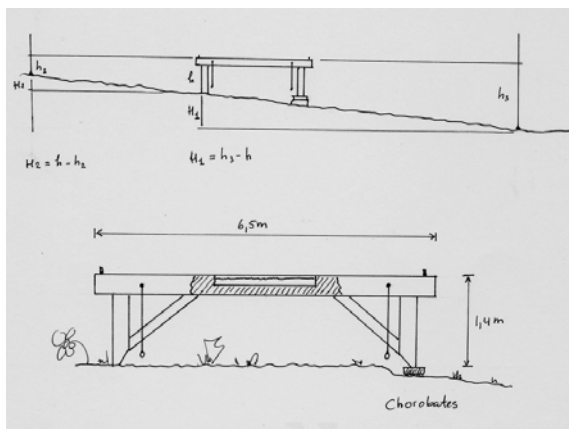
Fig 3 : représentation schématique du Chorobate
