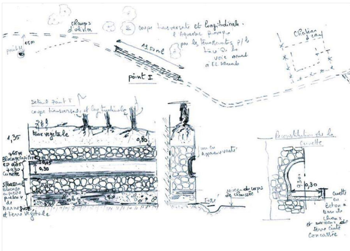
Fig 4. 47: Représentation en longitudinale et transversale du tronçon points 25-26 Source : Auteurs
