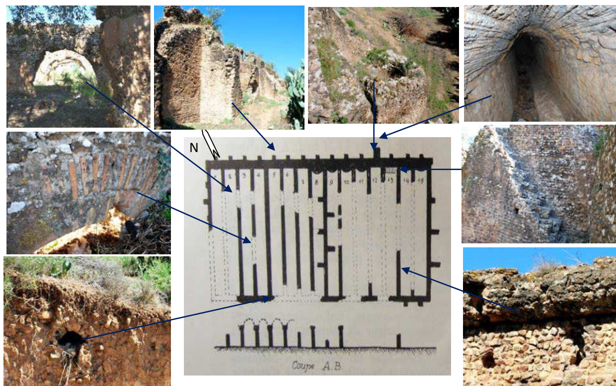
Fig.3.6 : Plan des citernes et photos associés aux éléments de composition : contrefort extérieur, puits, escalier d'accès au puits de puisage et jaugeage, système constructif, aqueduc tunnel de distribution, et aboutissement aqueduc de Fenaia
