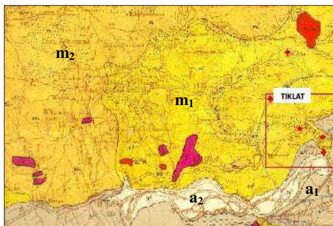
Fig 1.12: Géologie de la région de Fenaia
