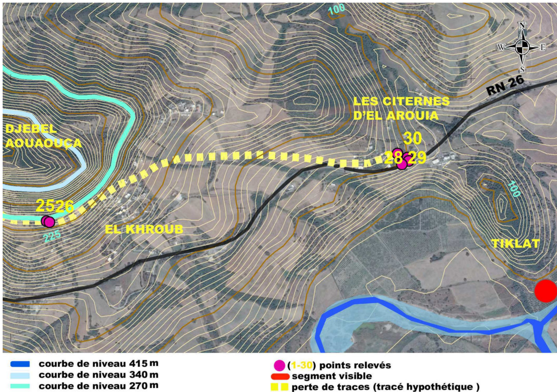
Fig 4. 53 : Carte représentant le tracé de l'aqueduc sur la troisième zone définie d' El Kharroub aux citernes d'El Ariouia Source : Auteurs
