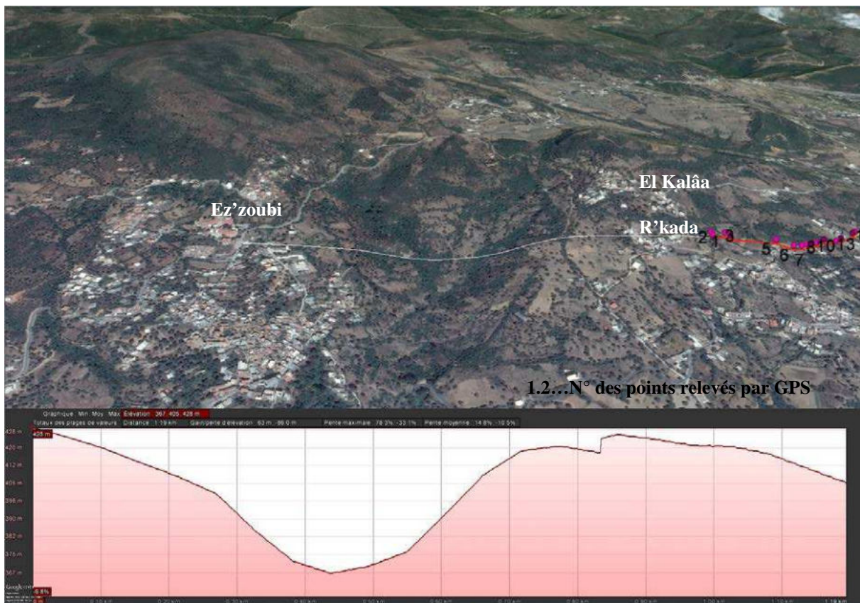
Fig. 4.15 : Représentation en profil/image aérienne de la dépression entre le village de Z'zoubia et R'kada (Thala Itchouren) montrant une rupture physique entre les deux sites
