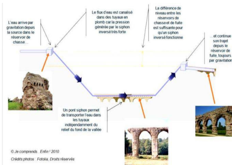
Fig 2. : Vue sur le système de fonctionnement de l'aqueduc siphon (sur pont et inversé), l'exemple du Gier
